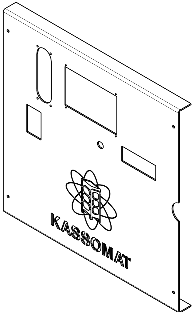
Isometrische Ansicht
