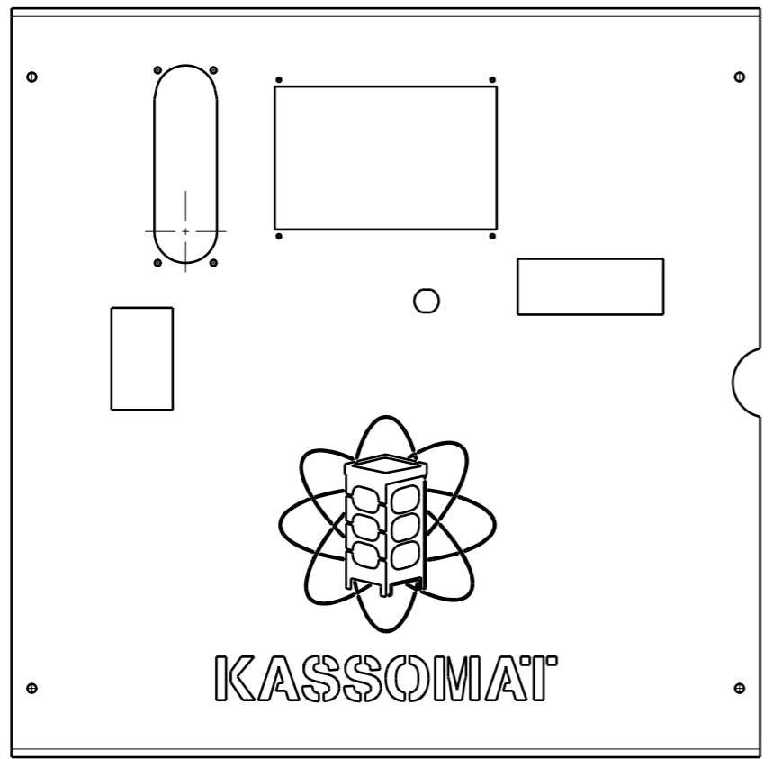
Vorderansicht
