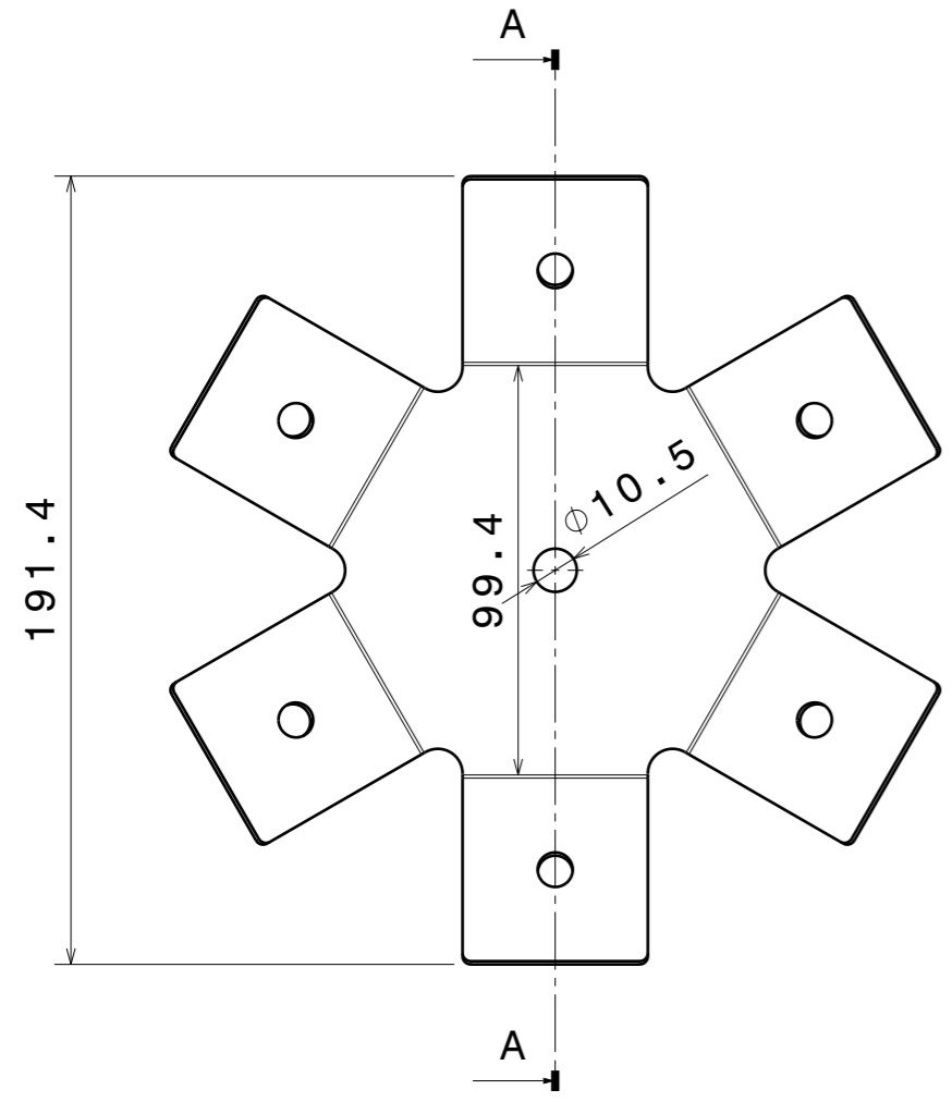
Vorderansicht
