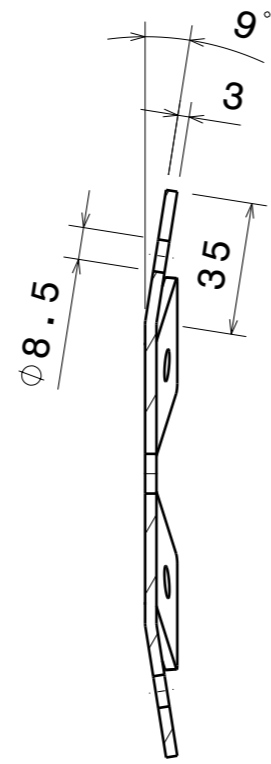
Schnittansicht A-A
