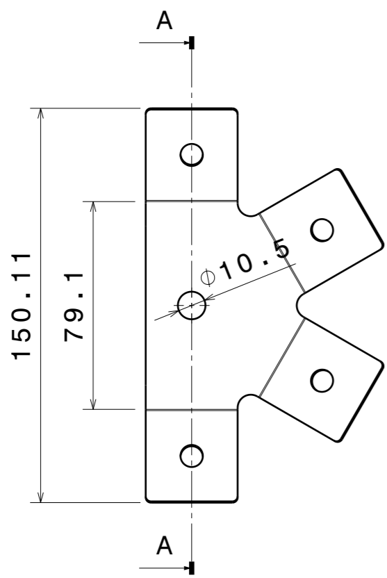
Vorderansicht
