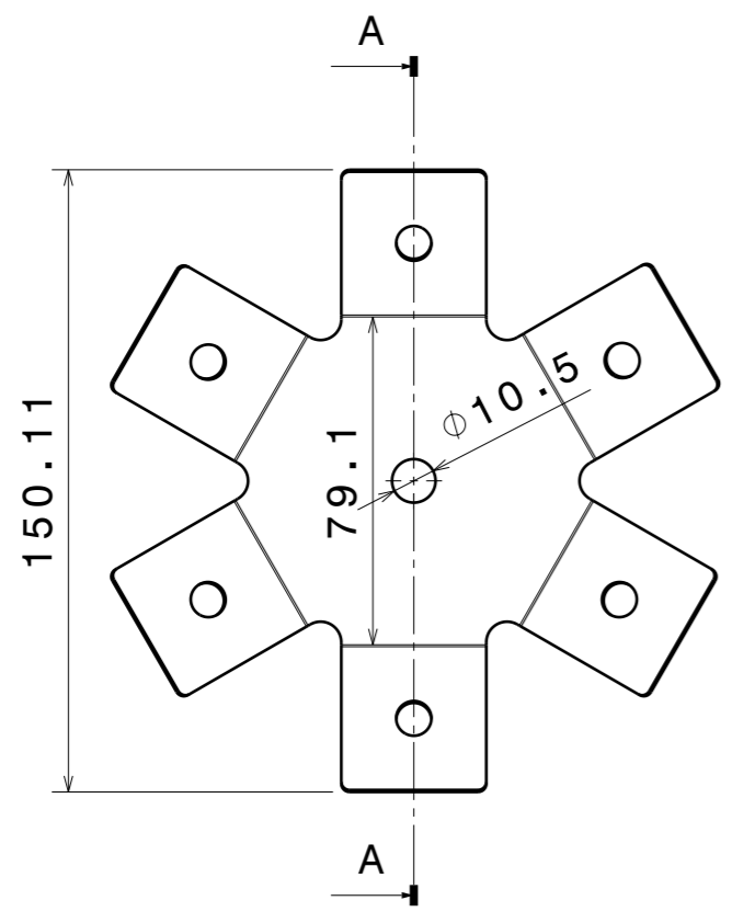
Vorderansicht
